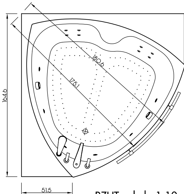
RZUT - skala 1:10
