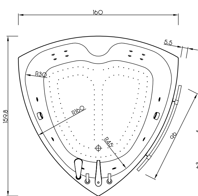
RZUT - skala 1:10
