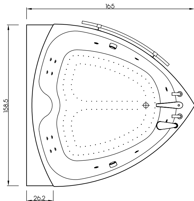
RZUT - skala 1:10
